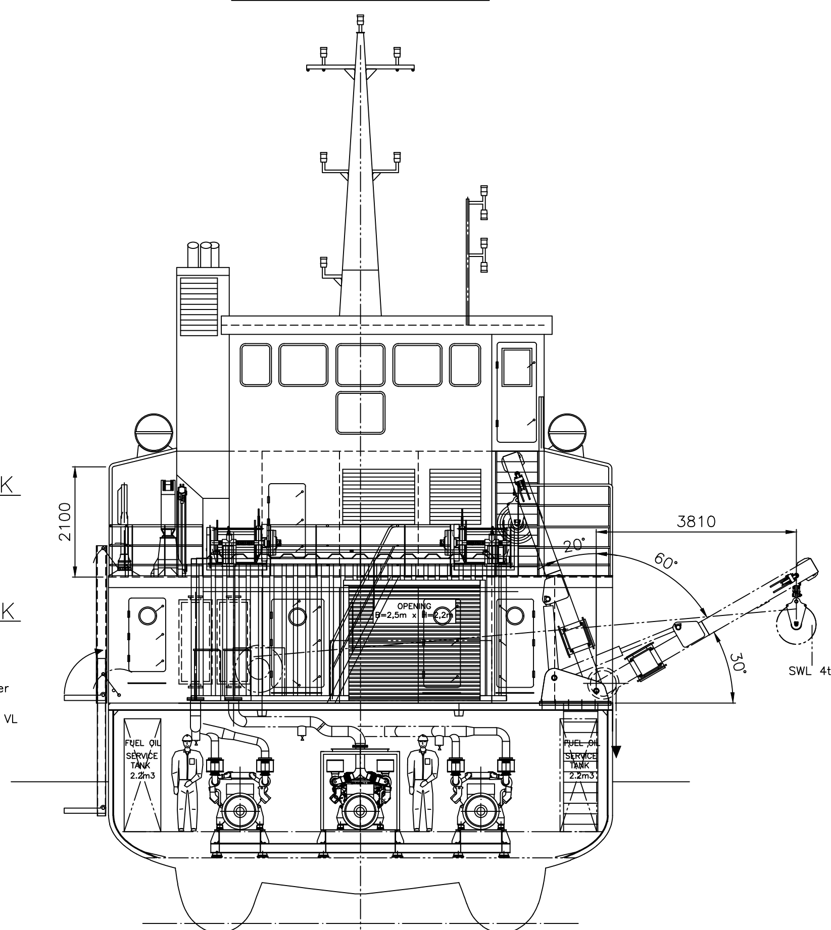
SECTION FR.17
